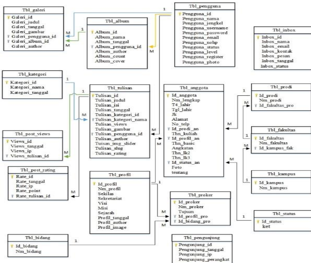
Gambar 3.4 Skema Tabel
