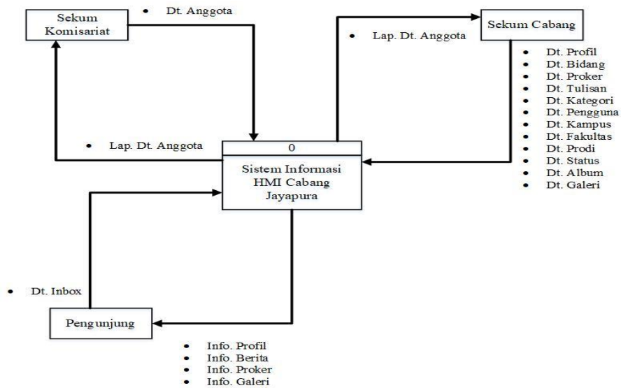
Gambar 3.1 Diagram Konteks
