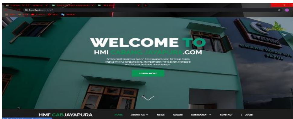
Gambar 4.1 Menu Utama
