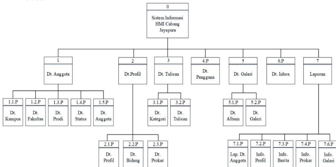
Gambar 3.2 Diagram Berjenjang
