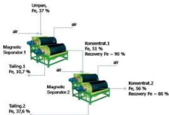
Gambar 1. Separator trap megnetit
