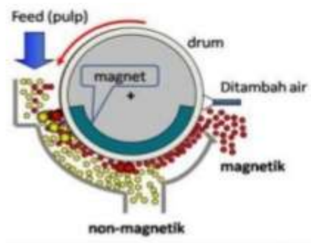
Gambar 5. Simulasi drum magnetit separator
