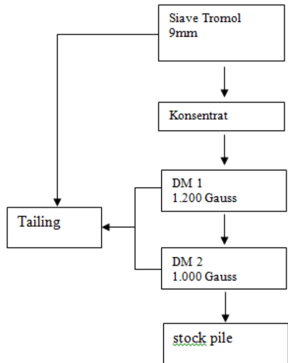
Gambar 6. Proses kerja pada magnetit separator
